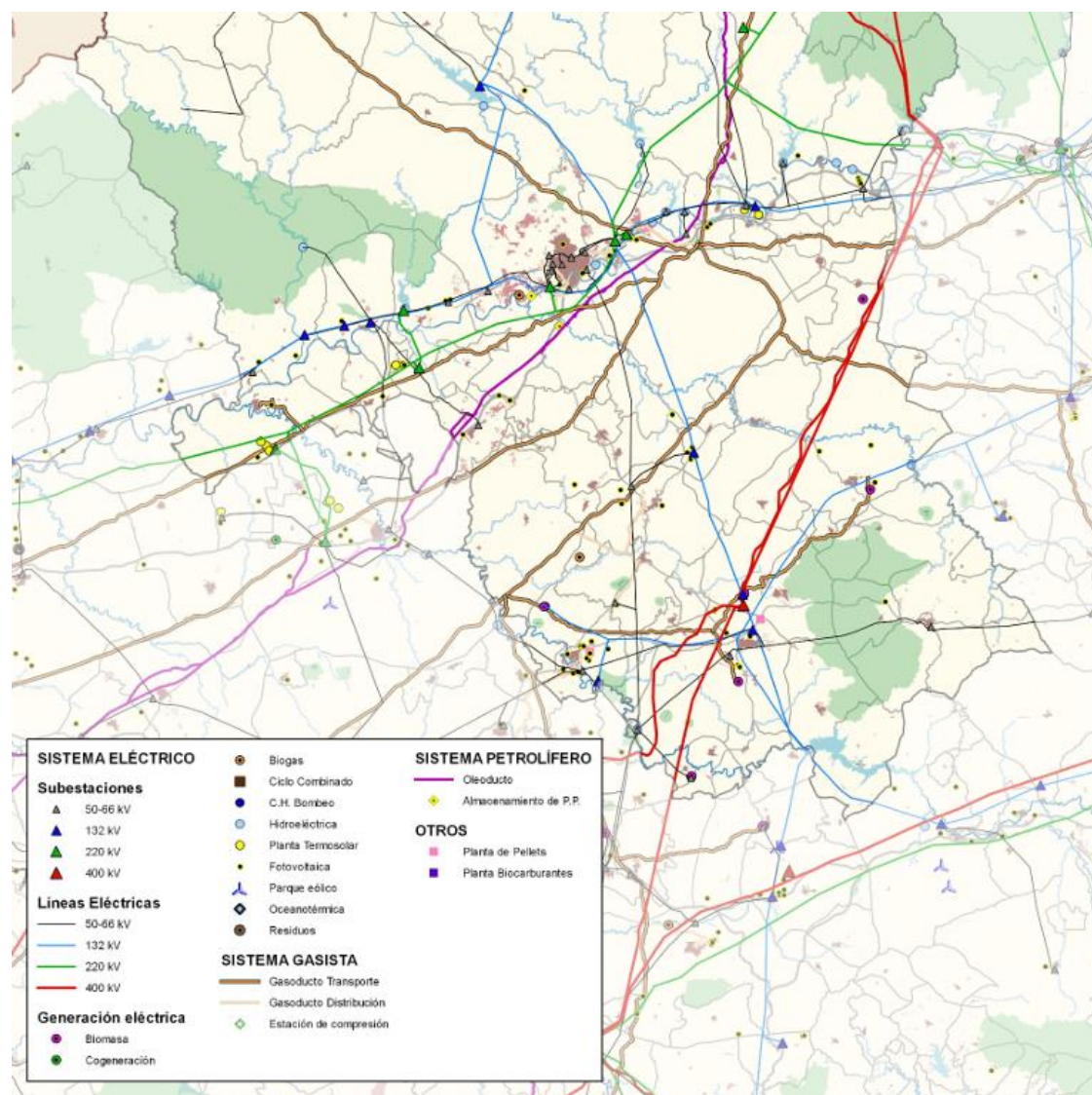
Mapa 4. Mapa 3. Infraestructuras energéticas
